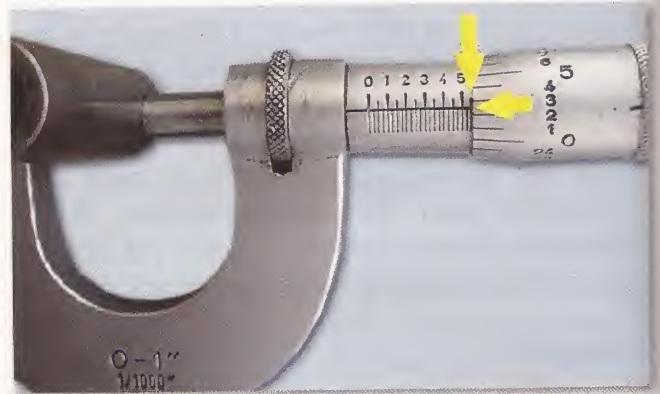
Micrómetro manual
